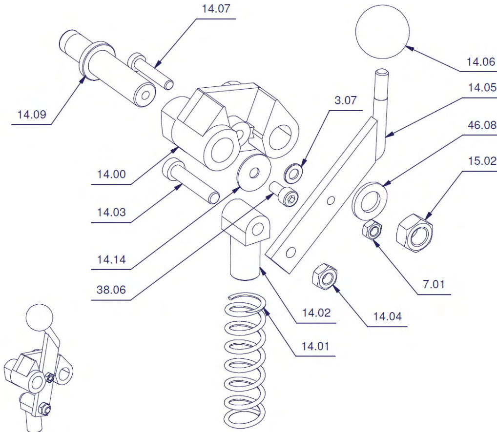
14.41 Spannwalzenhalter kpl./ Roller clamp compl.
